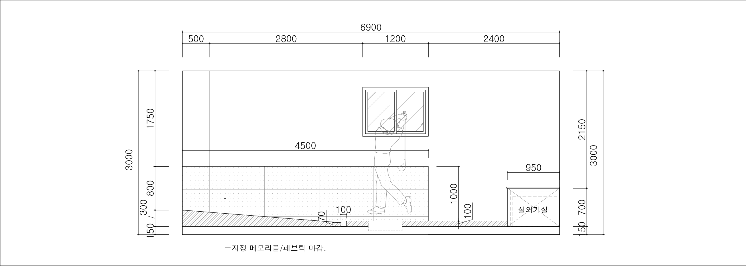
ELEVATION 'D'
