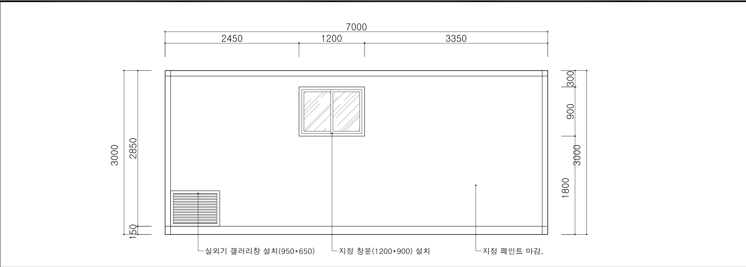
ELEVATION 'C'
