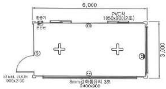
평면도
