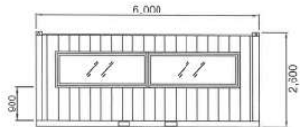
정면도
